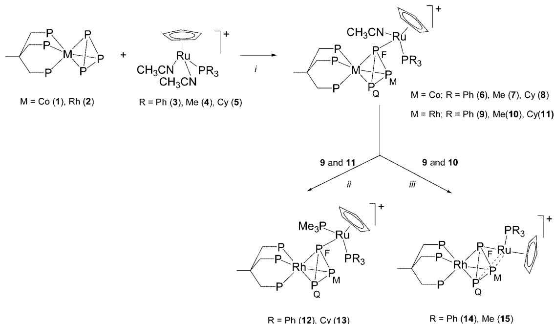
Scheme 2. i) CH 3 CN, CH 2 Cl 2 , toluene; ii) CH 2 Cl 2 , PMe 3 , toluene; iii) CH 2 Cl 2 , toluene.
